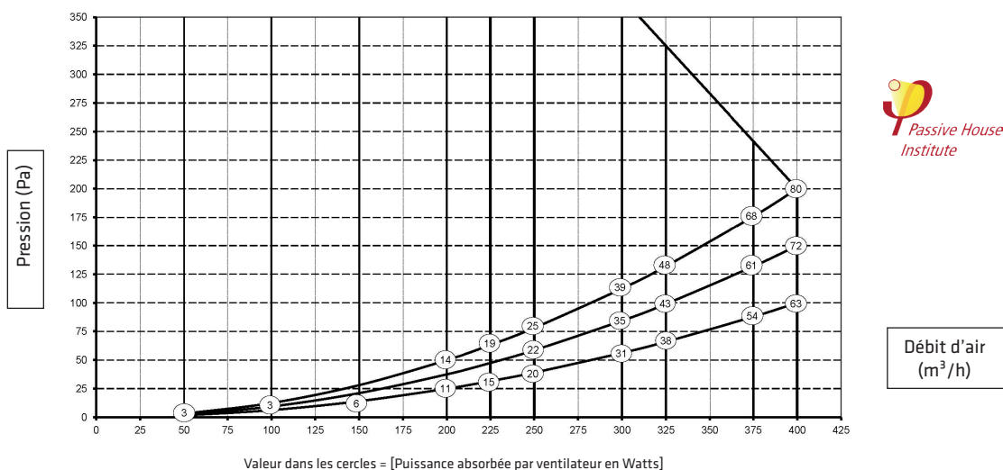
Diagramme débit (m³/h) / Pression (Pa) FLAIR 400
