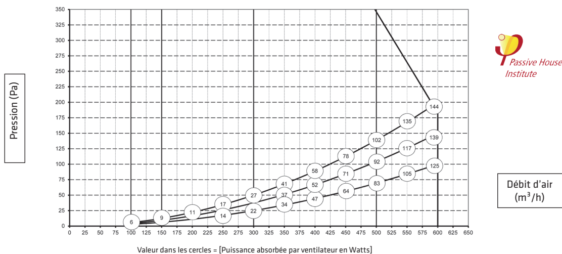
Diagramme débit (m³/h) / Pression (Pa) FLAIR 600
