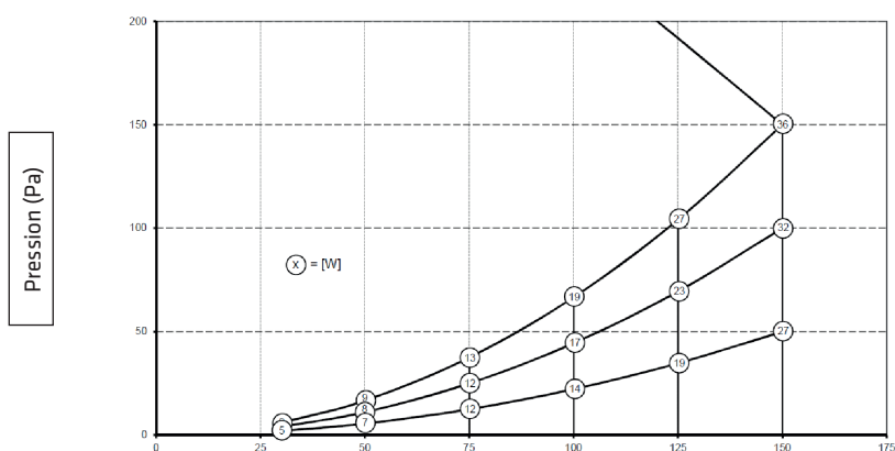
Diagramme débit (m³/h) / Pression (Pa) Renovent Sky 150 / 150+
