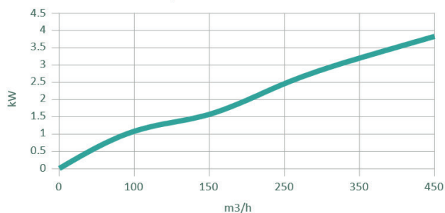
Puissance thermique G-4000 hiver [kW] Température air neuf extérieur -22°C
