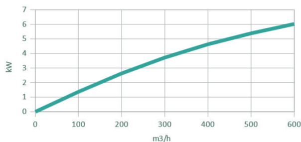
Puissance thermique G-6000 été [kW] Température air neuf extérieur 35°C
