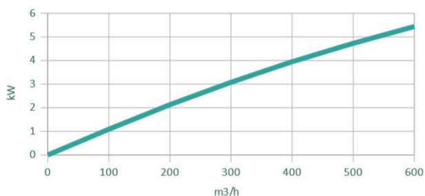
Puissance thermique G-6000 hiver [kW] Température air neuf extérieur -22°C
