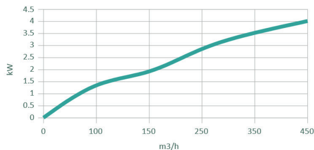
Puissance thermique G-4000 été [kW] Température air neuf extérieur 35°C
