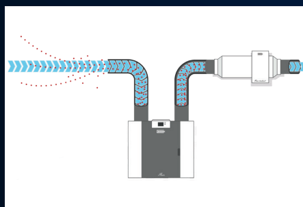
Pure induct Installation sur la gaine d'air neuf
