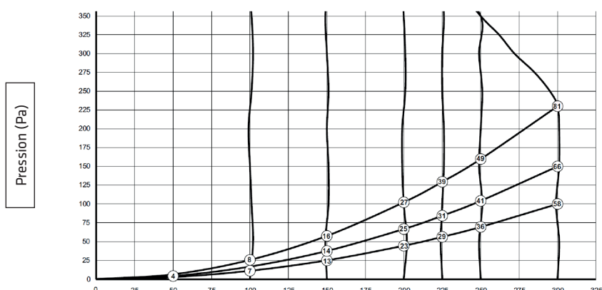
Diagramme débit (m³/h) / Pression (Pa) Renovent Sky 300 / 300+
