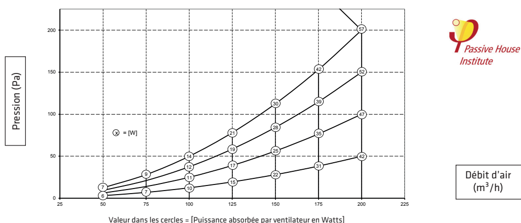
Diagramme débit (m³/h) / Pression (Pa) Renovent Sky 200 / 200+
