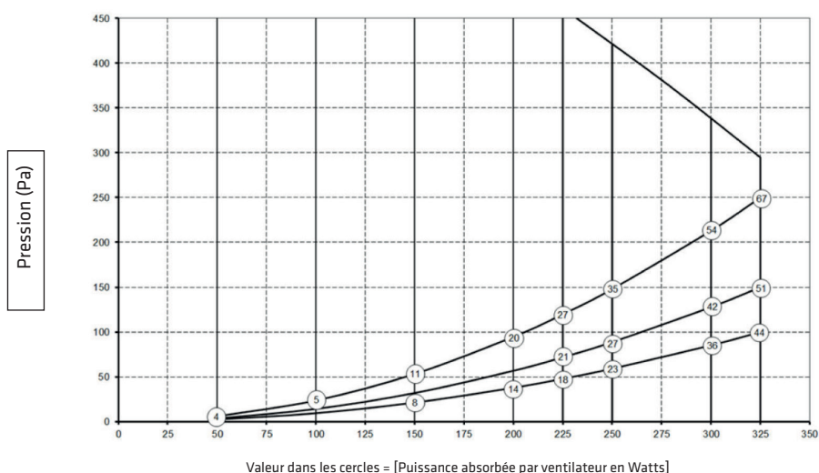
Diagramme débit (m³/h) / Pression (Pa) FLAIR 325
